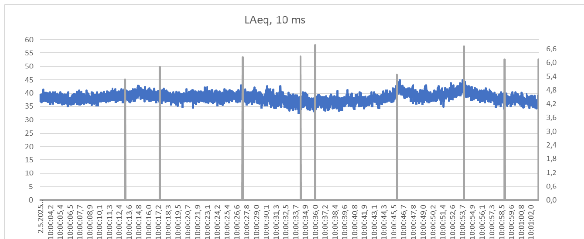
Kuva 3.1 Tallenteen 16 kuvaaja (sininen) ja iskumaisuutta kuvaava kerroin P ajan suhteen (harmaa). Tapahtuma on iskumainen, jos kerroin P > 6,6 dB. Iskumaisia tapahtumia havaitaan 2 kpl. Tallenteen signaalille ei ole tehty mittausselvitys-, taustamelu-, eikä tuulisuojakorjauksia.
