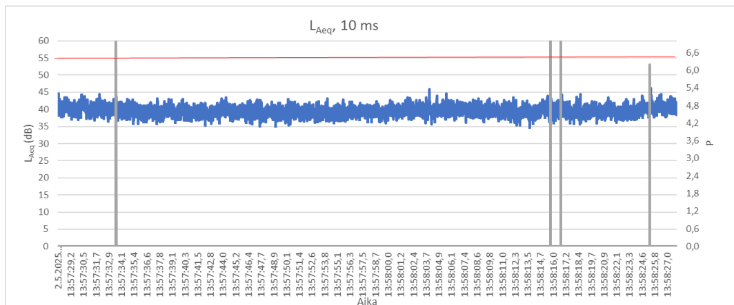
Kuva 3.1 Tallenteen 44 kuvaaja (sininen) ja iskumaisuutta kuvaava kerroin P ajan suhteen (harmaa). Tapahtuma on iskumainen, jos kerroin P > 6,6 dB. Iskumaisia tapahtumia ( P > 6,6 dB) havaitaan 3 kpl. Tallenteen signaalille ei ole tehty mittauslevy-, taustamelu-, eikä tuulisuojakorjauksia.
