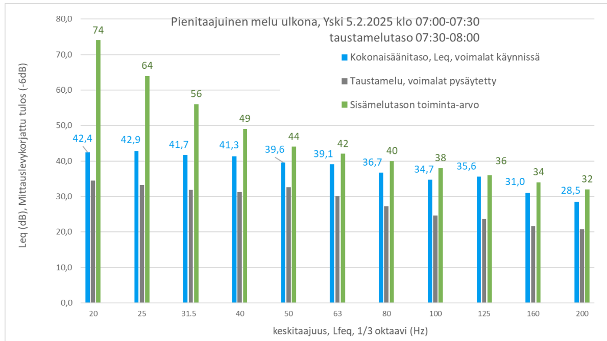
Kuva 1: Pienitaajuinen melu (taajuuskorjaamaton ekvivalenttiäänitaso, L_{eq} , taajuuudet 20-200Hz), Yski 5.2.2025 klo 7:00-7:30.
