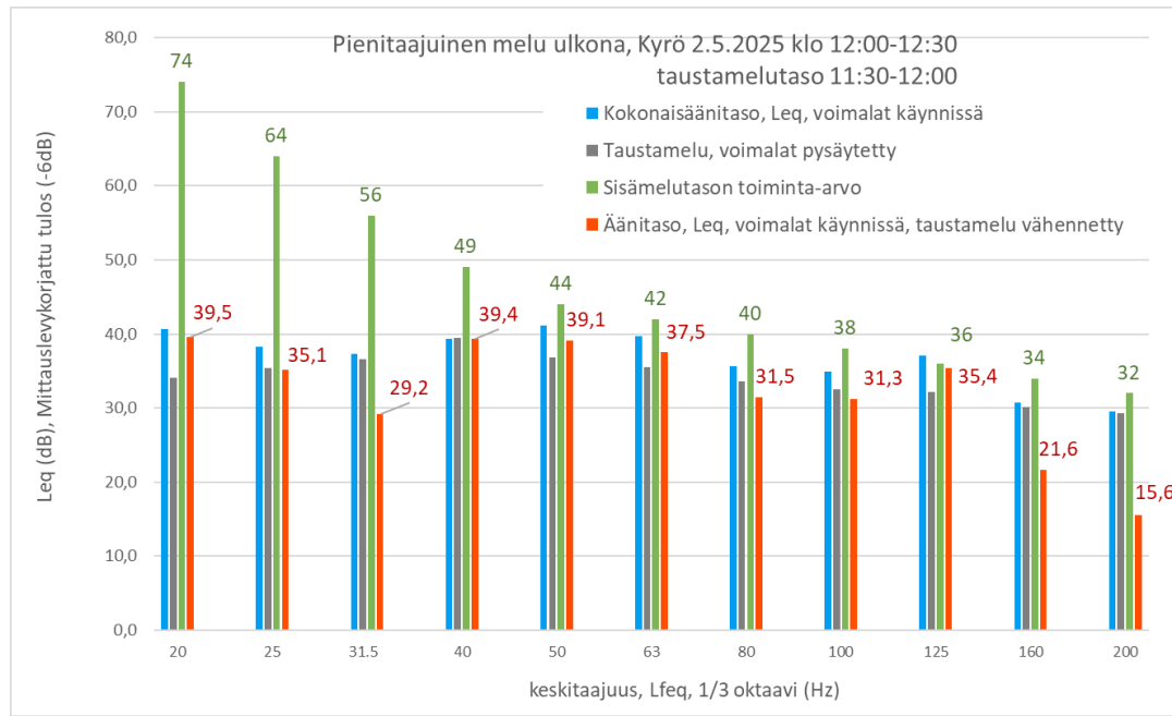
Kuva 1.1: Pienitaajuinen melu (taajuuskorjaamaton ekvivalenttiäänitaso, L_{eq} , taajuudet 20-200Hz), Kyrö 2.5.2025 klo 11:30-12:30. Taustamelutaso ylitti melutason voimaloiden käydessä 40 Hz terssitaajuudella, joten sitä ei ole vähennetty äänitasosta ko. 40 Hz taajuuskaistalla.
